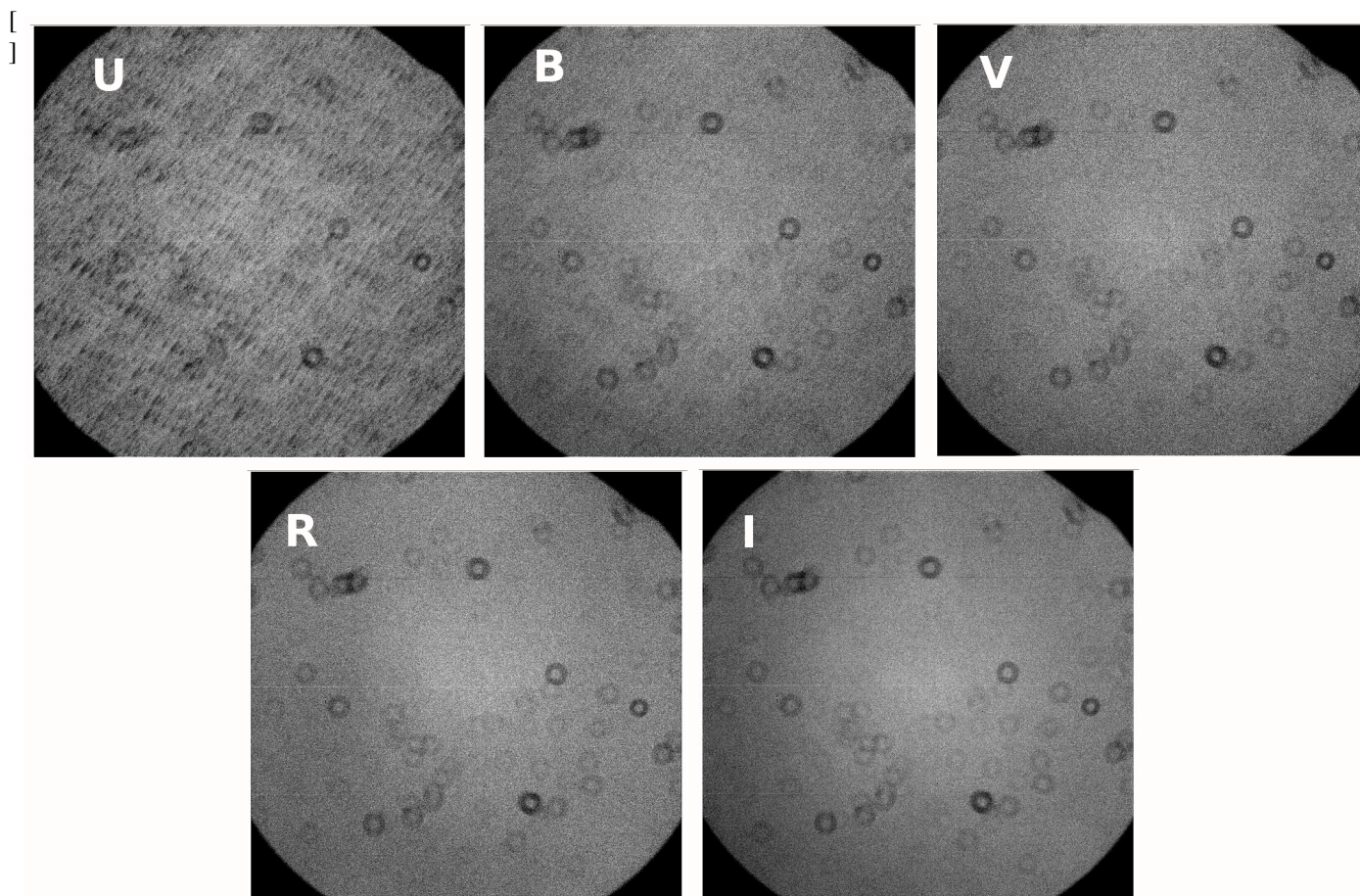
Figura 6. Imágenes de campos planos en los filtros UBVRI de la rueda Italiana. Las pequeña donas que se pueden observar en todas las imágenes se deben a polvo en la ventana del criostato.
