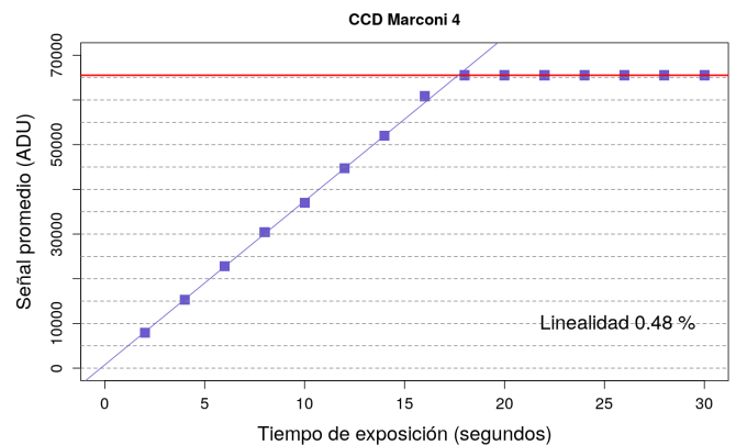
Figura 2. Gráfico de linealidad del CCD-M4
