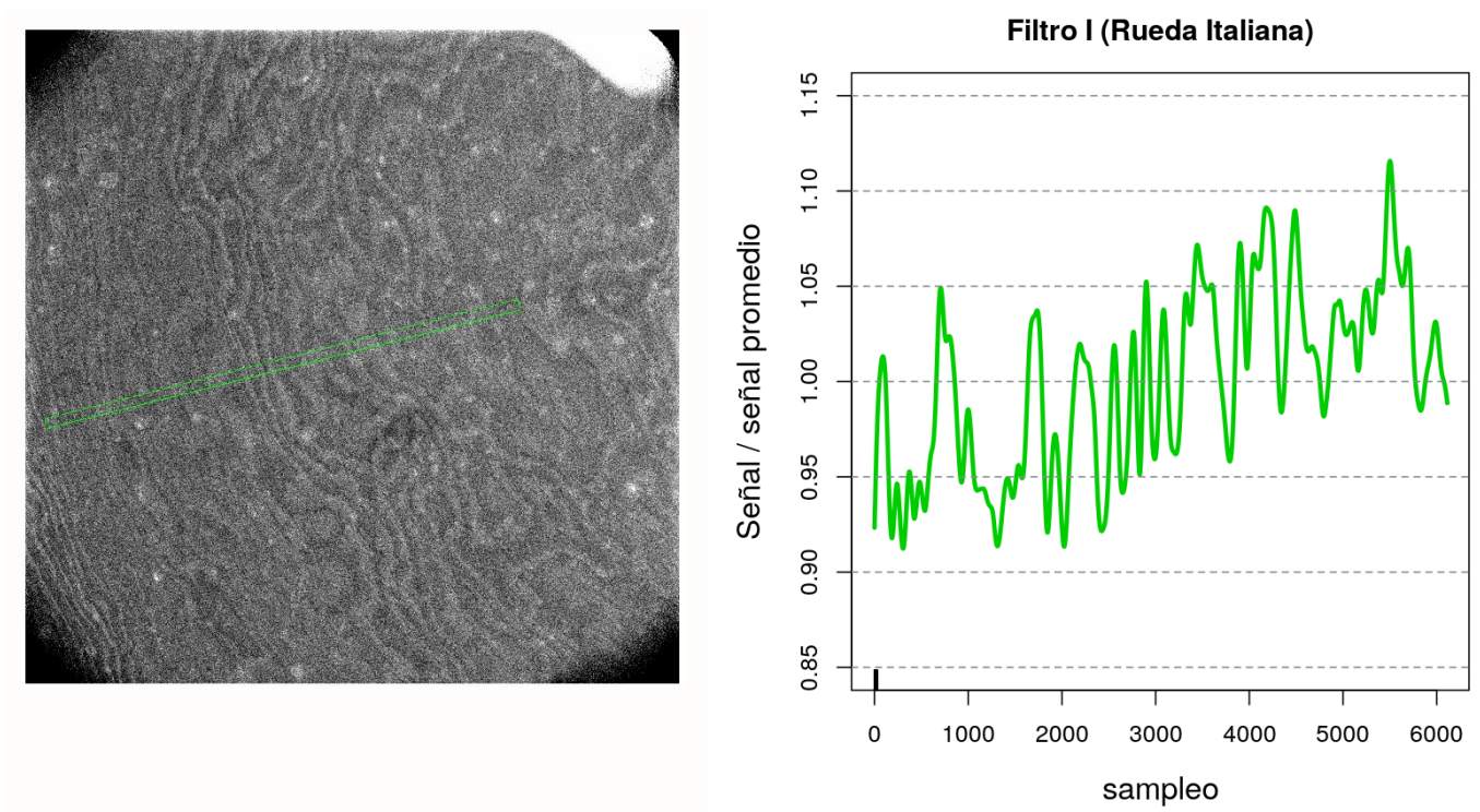
Figura 7. Patrón de franjas de interferencia en el filtro I con el CCD-M4 y gráfico de la amplitud de las mismas.
